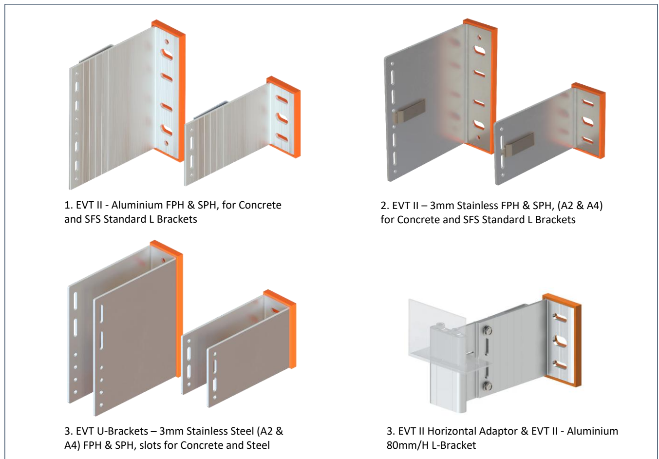
EVT II wall bracket examples.
